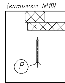
Крепление дна ящика (комплект №10)
