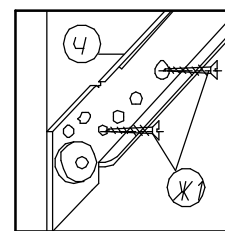
Крепление роликовой направляющей (комплект №25) левая
